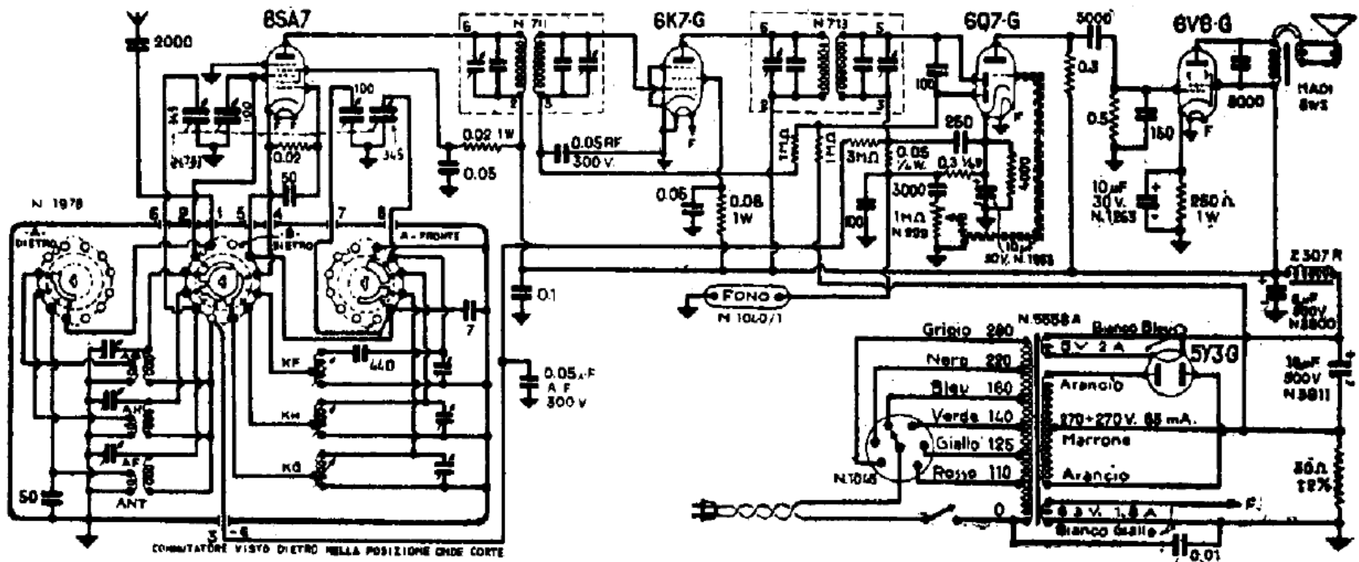
RICEVITORE SUPER G.72 S
